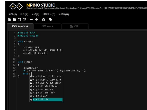
[ 아두이노 C언어 ]
